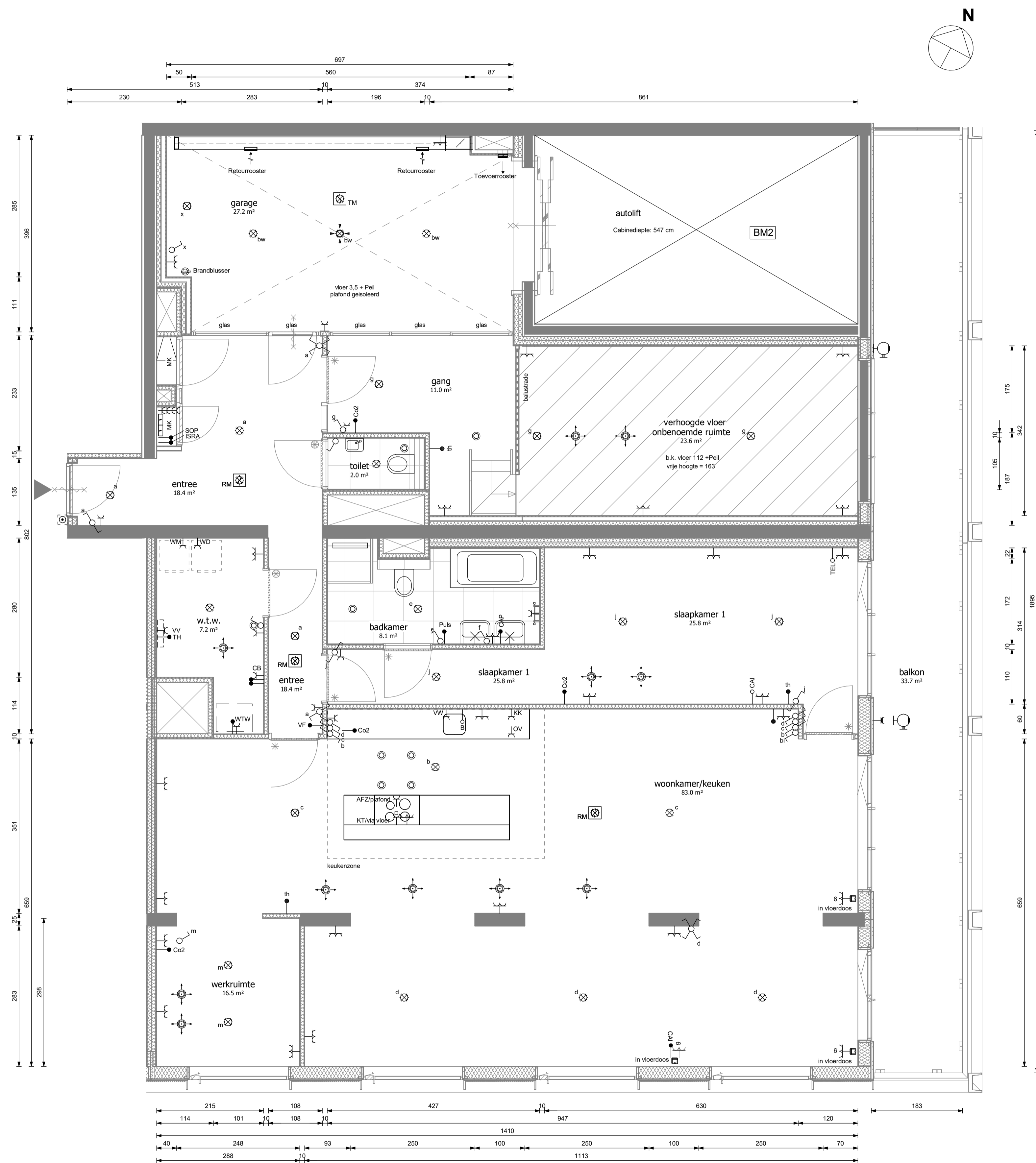
Type C7b schaal 1 : 50
