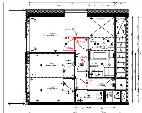
Eerste verdieping type A1asp
